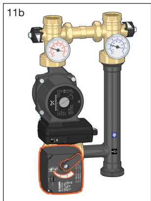
Versione HE2 Pompa UPML 25-105
