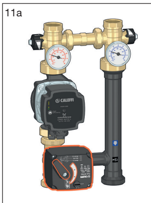
Versione HE1 Pompa UPM3S Auto 25-60
